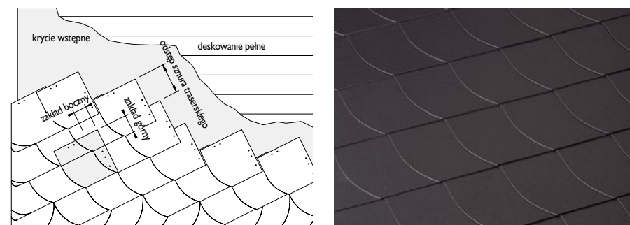
Przykład: Format 30 x 30 cm, ze zintegrowaną stopą i początkiem krawędzi
