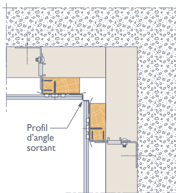
Avec isolant
