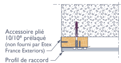
Sans isolant
