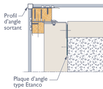
Avec isolant
