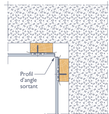
Sans isolant
