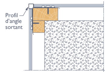
Sans isolant
