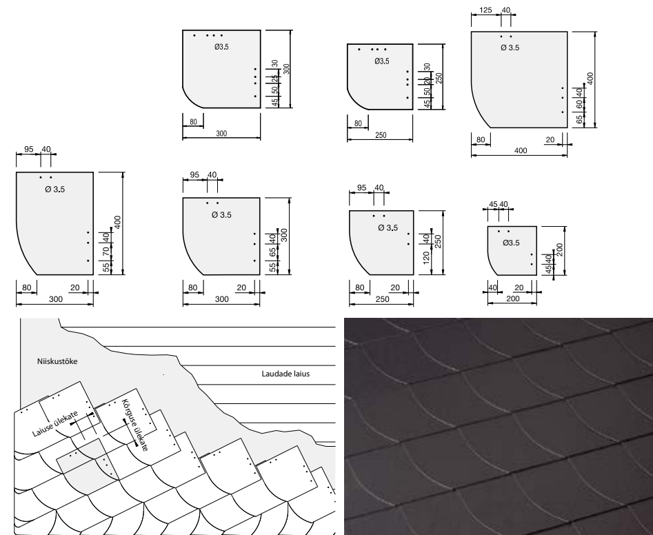
Näide: 30 × 30 cm saksapärane kate
