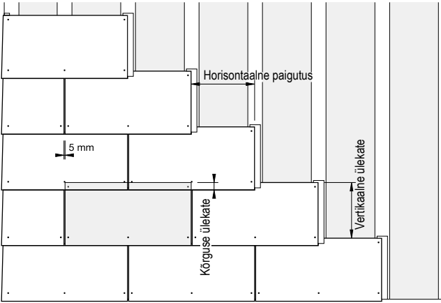
Näide: 60 × 30 cm fassaadiplaatide ristkülikukujuline kate
