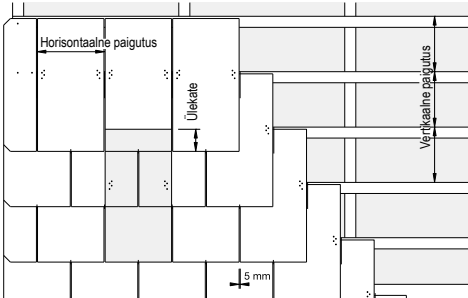
Näide: 30 × 60 cm topeltkate
