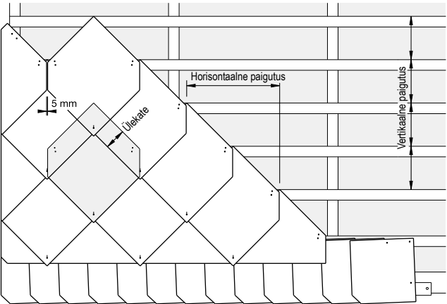
Näide: 40 × 40 cm teravaservalise rombi kate 30 × 30 cm komplektiplatidega
