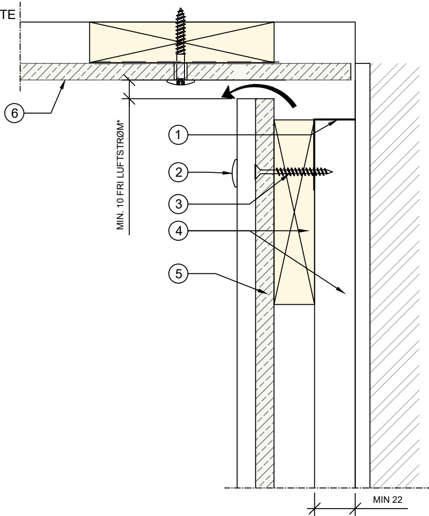
SEKTION 1:2
