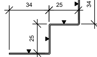
INVENDIGT HJØRNE PROFIL
