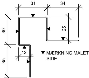
ASYMMETRISK UTVENDIG HJØRNE PROFIL
