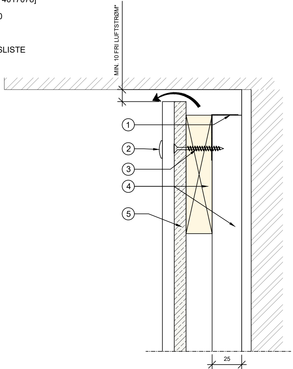
SEKTION 1:2
