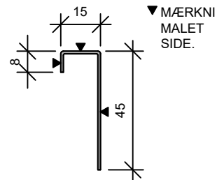
ENKEL ENDEKANT PROFIL
