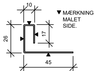
DOBBELT ENDEKANT PROFIL
