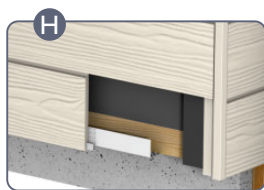
H Profil wentylacyjny perforowany 50x30x2500mm lub 70x30x2500mm lub 100x30x2500mm
