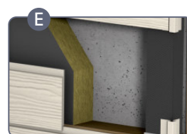
E Taśma uszczelniająca PCV 100x0,5mm L=30m
