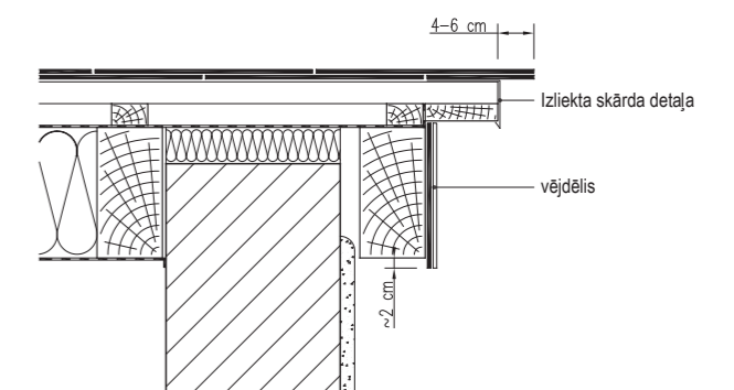
Vējmalas ierīkošana, izmantojot "Cedral" jumta plāksnīti
