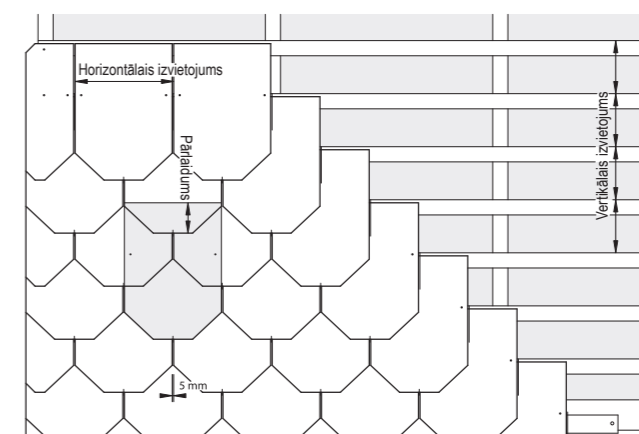
32 x 45 cm dubultais klājums
