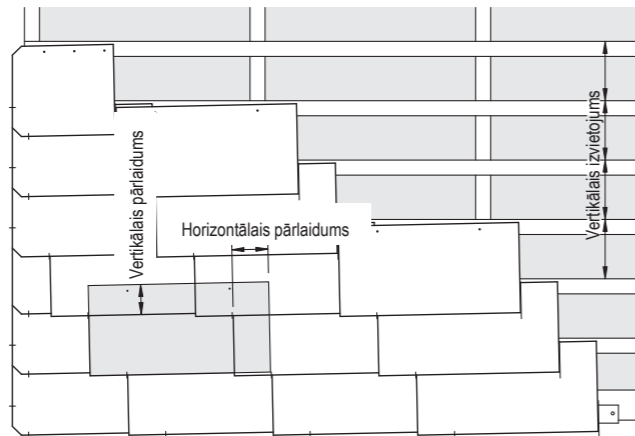
Horizontālais klājums, izmantojot 60 x 30 cm formāta plāksnītes
