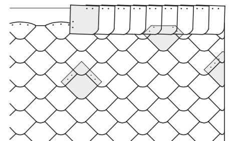
Fasādes augšējās daļas un malas ierīkošana ar uzklāšanas metodi
