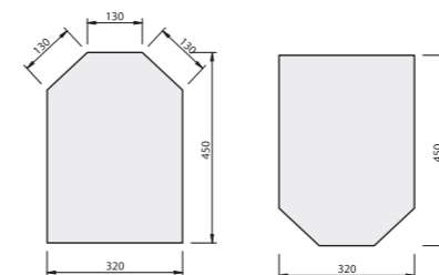
32 x 45 cm plāksnītes
