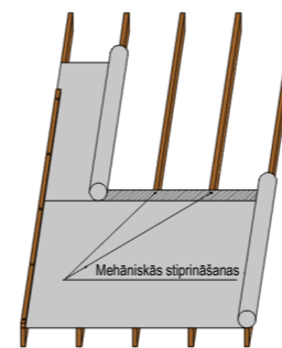
1 att. Stiprinājums pie spārēm
