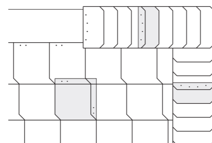
Fasādes augšējās daļas un malas ierīkošana, izmantojot 30 x 15 cm plāksnītes
