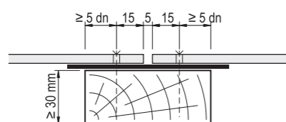
Savienojuma šuves ierīkošana dn – stiprinājuma skrūves šķērsriezums
