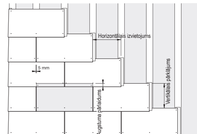
60 x 30 cm fasādes plāksnīšu taisnstūra klājums
