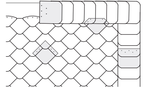
Fasādes augšējās daļas un malas ierīkošana ar pārlaiduma metodi
