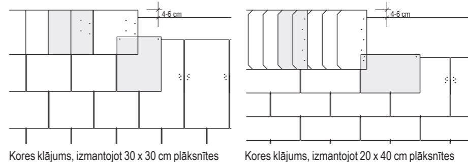
Kores klājums, izmantojot 30 x 30 cm plāksnītes, Kores klājums, izmantojot 20 x 40 cm plāksnītes
