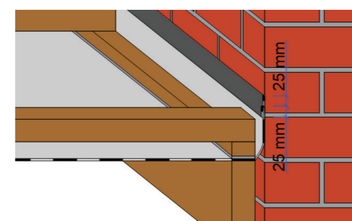
2 att. Difūzijas plēves stiprināšana pie sienas.
