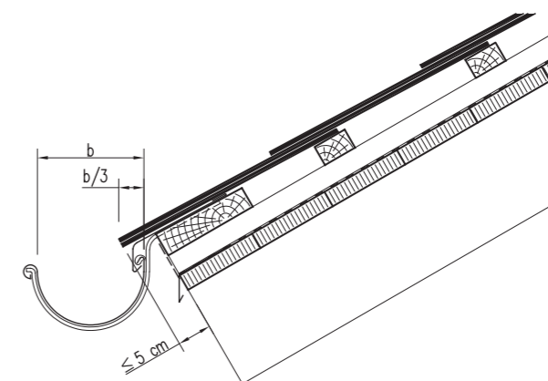
Teknes ierīkošana, klājot uz latām
