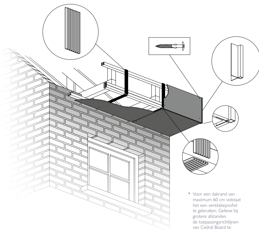
Ventilatieprofiel voor dakrand tot 60 cm* L= 3m PVC zwart
